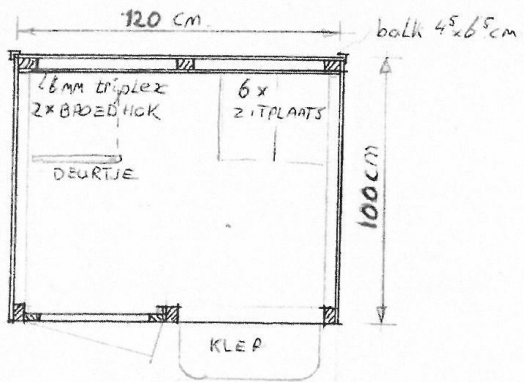
PLATTEGROND
