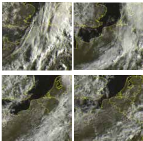
Afb. A, B, C en D Satellietbeelden 12 augustus 08:00, 11:00, 14:00 en 17:00 uur
