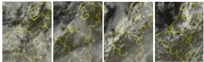
Afb. E, F, G en H Satellietbeelden 13 augustus 08:00, 11:00, 14:00 en 17:00 uur
