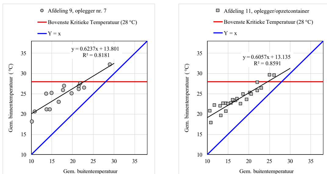
Figuur 2. De gemiddelde temperatuur in de wagen als functie van de gemiddelde temperatuur buiten. Links: voor het model duivenwagons van Afdeling 9 (meetgegevens afkomstig uit: Winkel & Van Stralen, 2012; Winkel & Van Stralen, 2013; Winkel & Van Iwaarden, 2018). Rechts: voor het model duivenwagons van Afdeling 11 (meetgegevens afkomstig uit: Heetkamp & Schrama, 2000; Heetkamp & Schrama, 2001; Heetkamp & Schrama, 2002). Elk bolletje/vierkantje in de figuren betreft een transport/vlucht. De meetgegevens betreffen alleen de perioden van het feitelijke rijden (exclusief pauzes en het verblijf op de losplaats).
